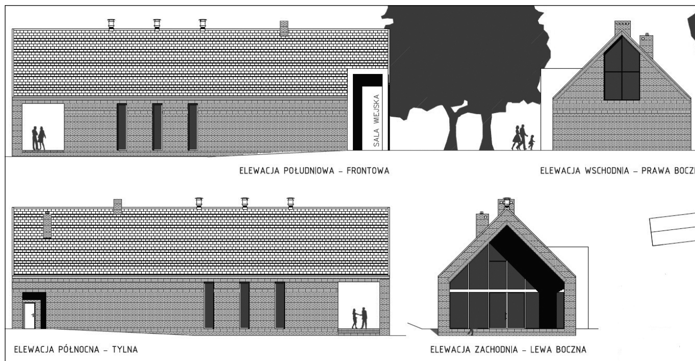
Elewacje Marianowo Herbutowo sala
