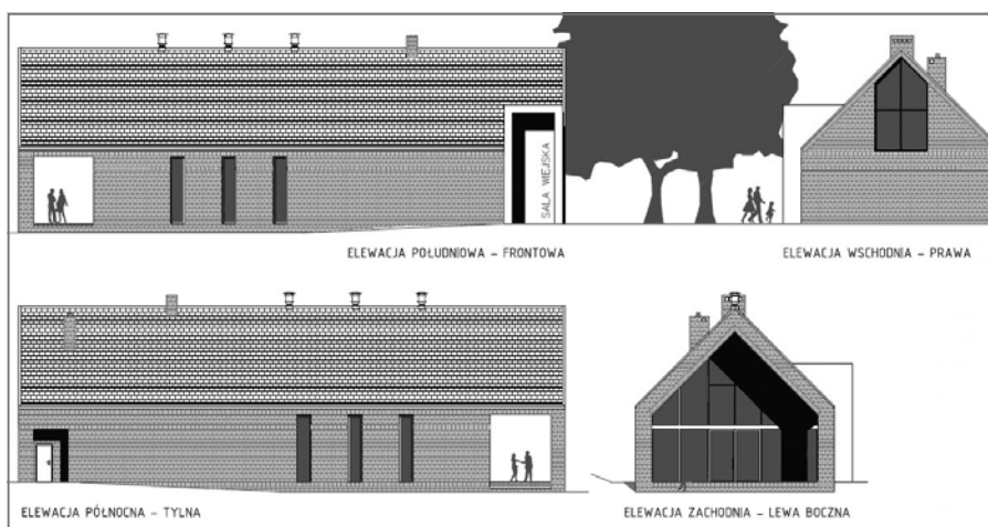
Wyciąg z projektu budowlanego sali wiejskiej dla sołectw Marianowo i Herburtowo
